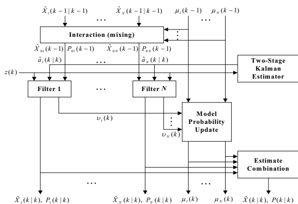
Fig. 1 AIMM algorithm.
